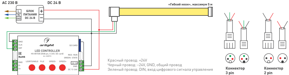
Схема 1. Подключение герметичной ленты «неон»
