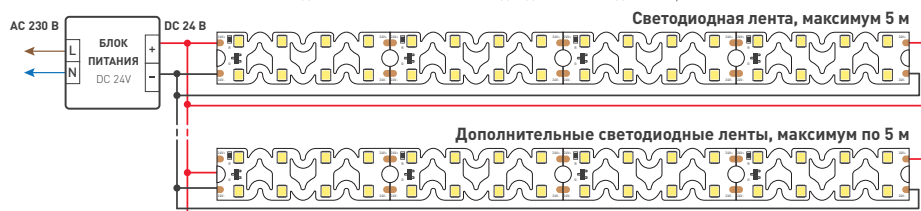
Схема 2. Подключение нескольких светодиодных лент с двух сторон для обеспечения равномерного свечения ленты по всей длине
